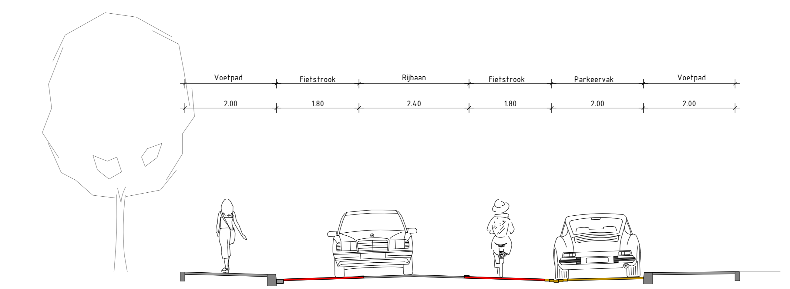
PROFIEL 1 NIEUWE SITUATIE LOOPAKKER SCHAAL 1 : 50
