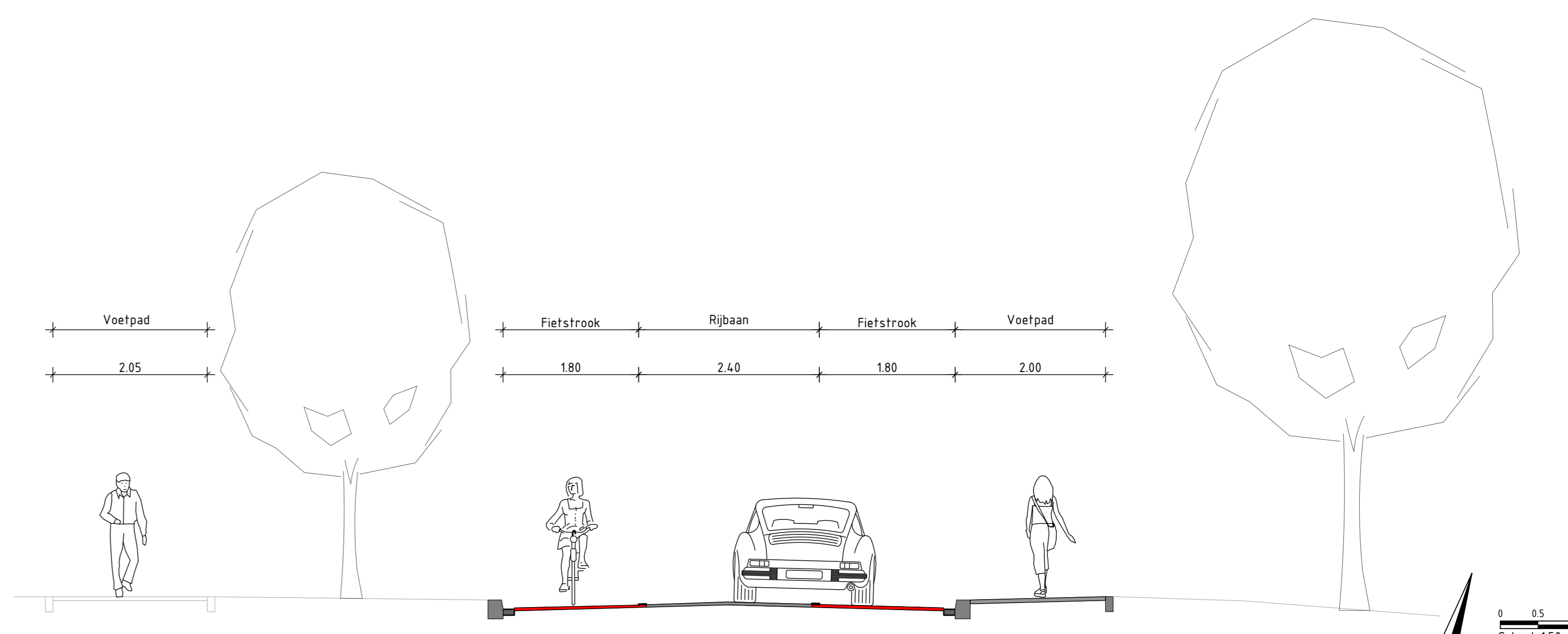
PROFIEL 2 NIEUWE SITUATIE VOORBURGGGRACHT SCHAAL 1 : 50
