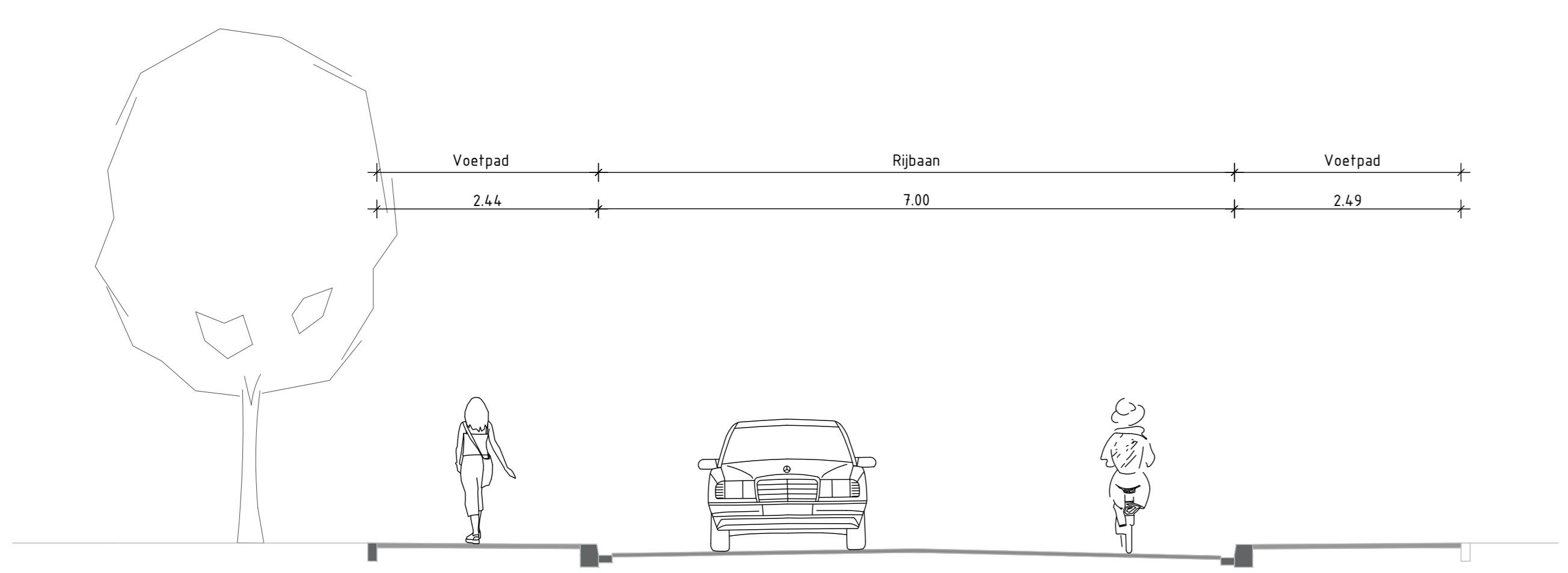
PROFIEL 1 BESTAANDE SITUATIE LOOPAKKER SCHAAL 1 : 50
