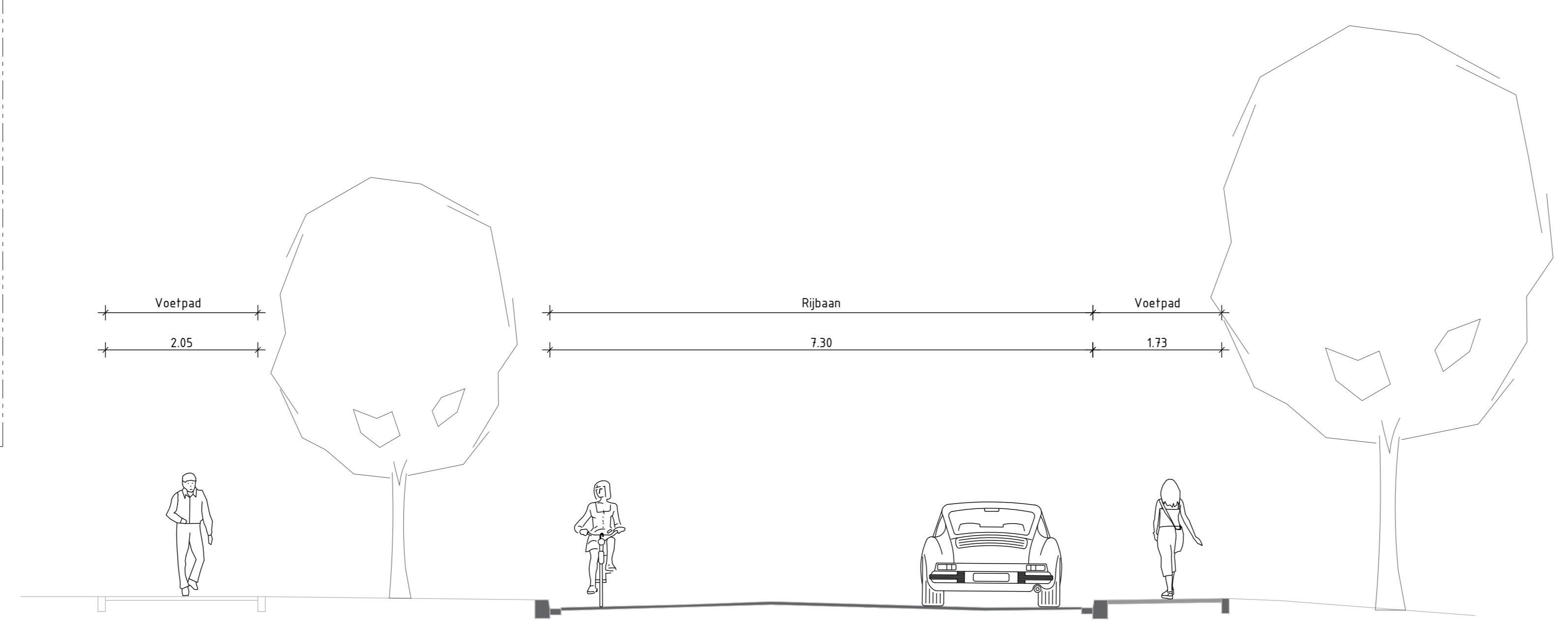
PROFIEL 2 BESTAANDE SITUATIE VOORBURGGGRACHT SCHAAL 1 : 50
