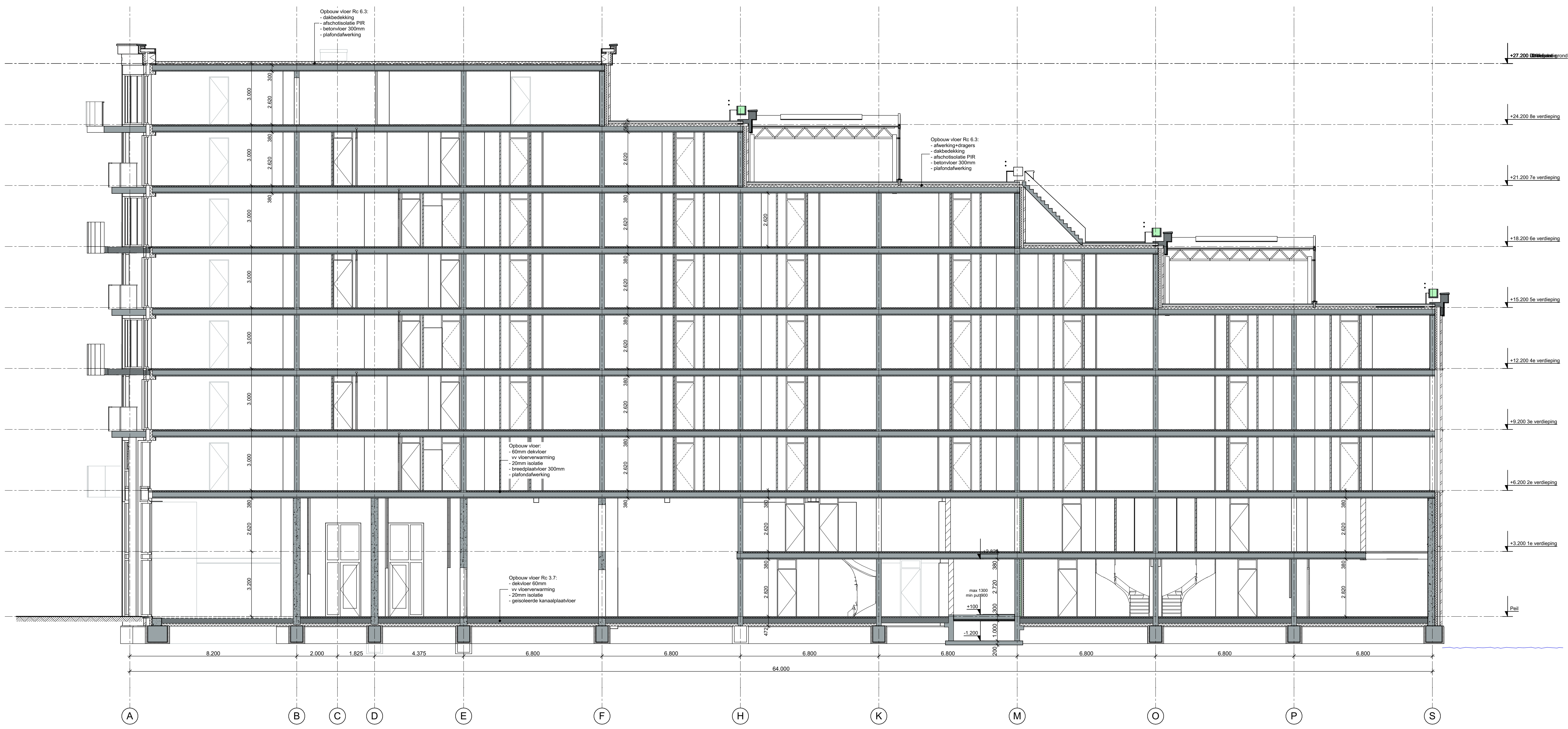
Doorsnede E-E Schaal 1:100
