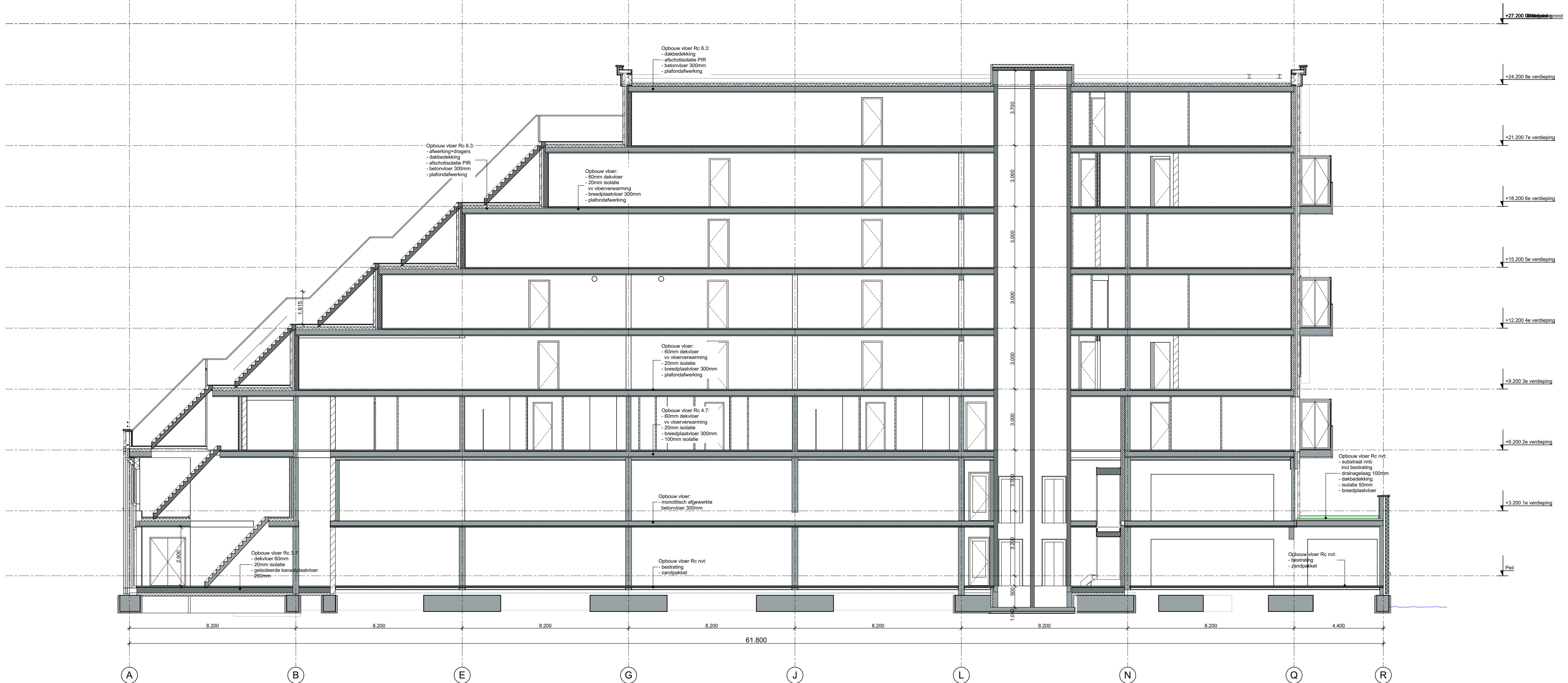
Doorsnede K-K Schaal 1:100
