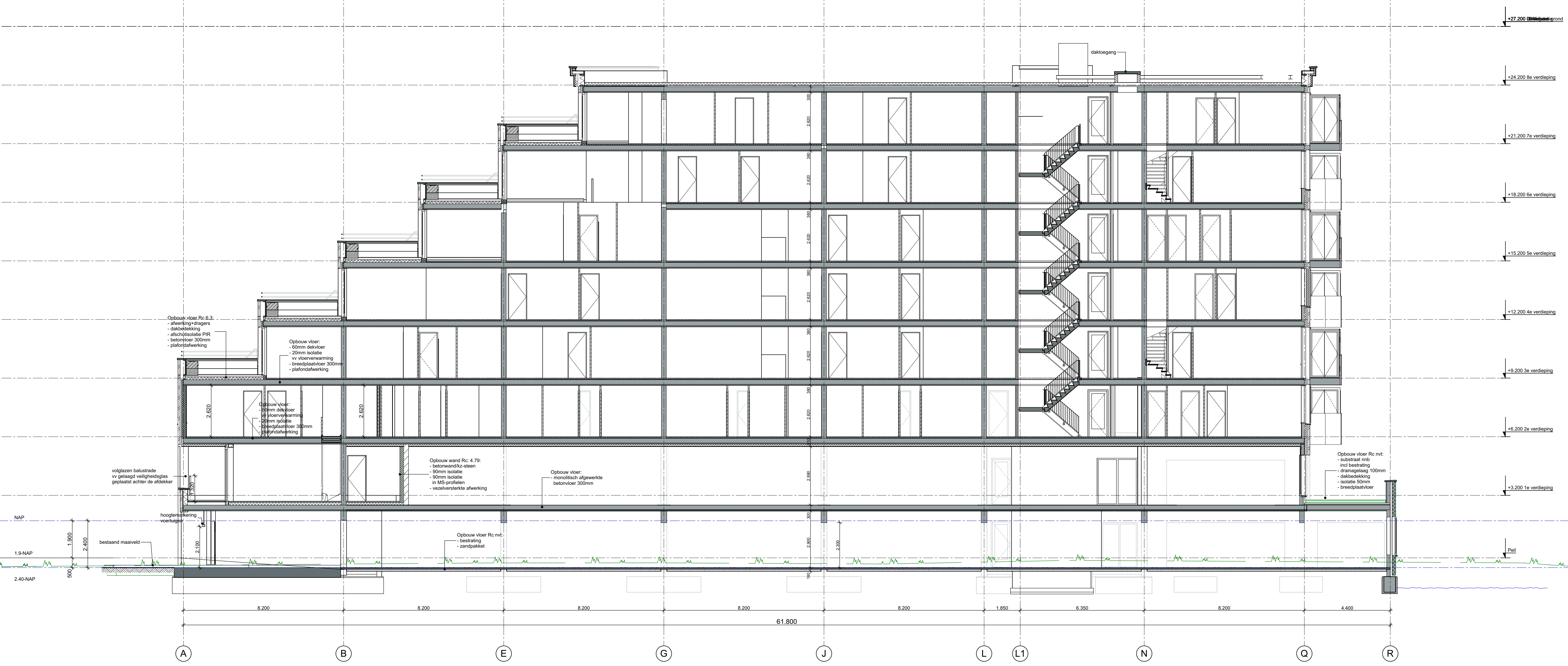
Doorsnede J-J Schaal 1:100
