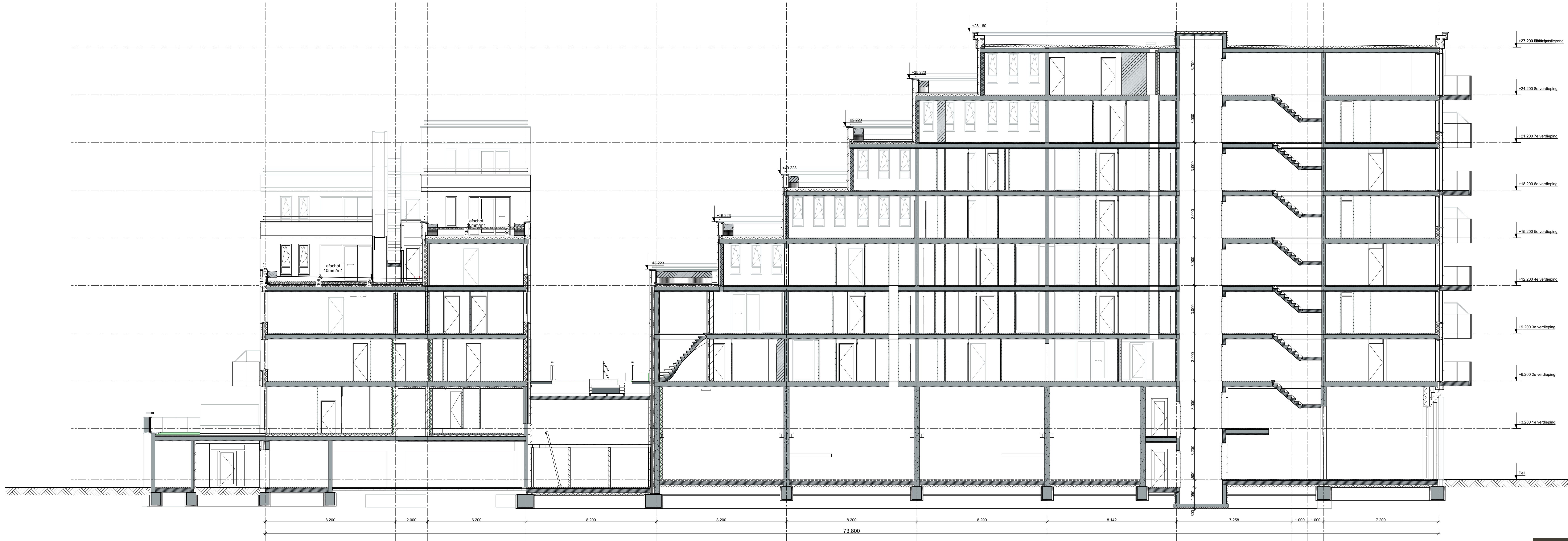
Doorsnede M-M Schaal 1:100
