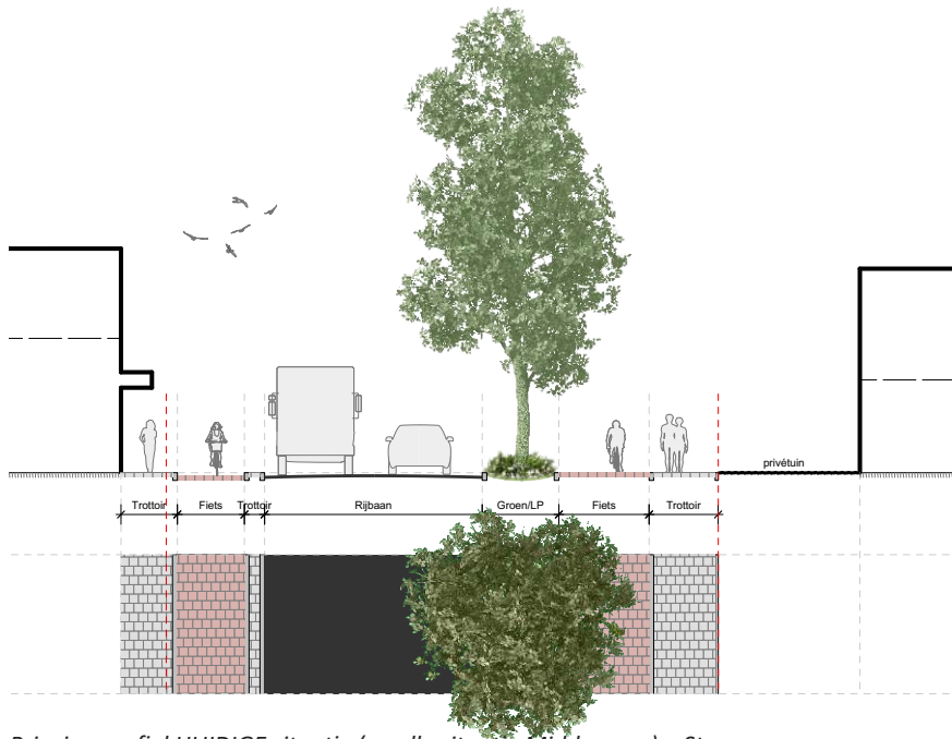
Principe profiel HUIDIGE situatie (smalle situatie Middenweg) – Stoep
